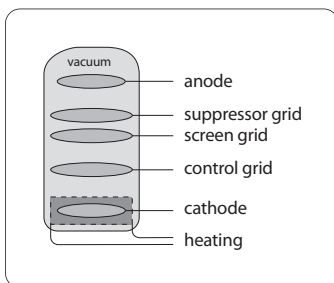
Fig. 1.5: pentode
